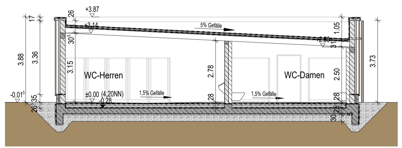
SCHNITT A-A
