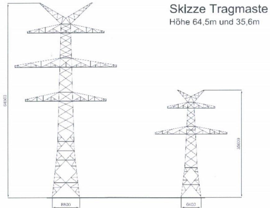
Abb. 2 Mastprinzipskizzen der möglichen Mastgestänge (nicht maßstabsgetreu)
