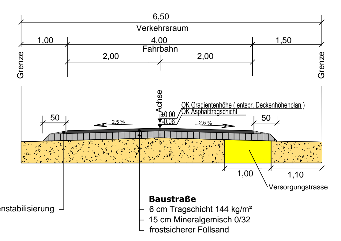
Schnitt B-B M. 1:50
