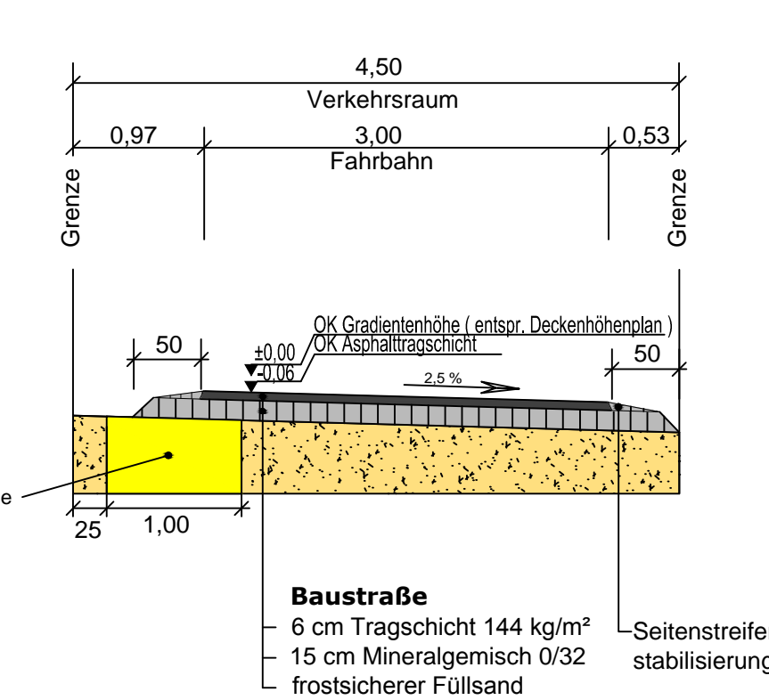
Schnitt B-B M. 1:50
