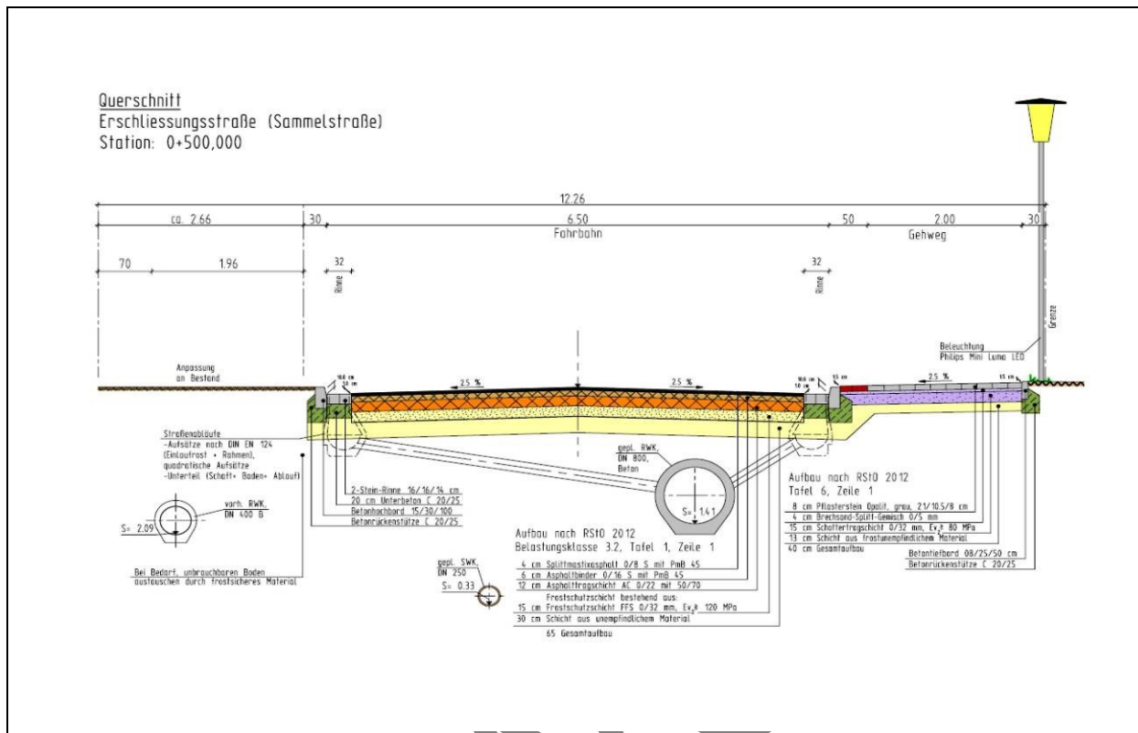
Abbildung 18: Regelquerschnitt Sammelstraße
